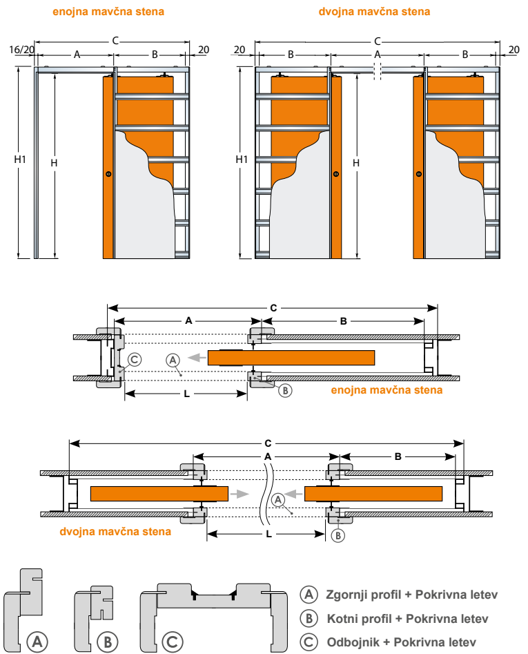
SHEMA PODBOJA VRAT ZA DRSNI SISTEM (sistem mavčnih sten)
